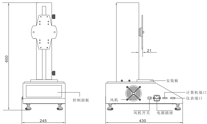
安装板尺寸
